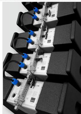
Auto-locking Flugvorrichtung.
