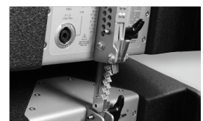
Auto-locking Flugvorrichtung.
